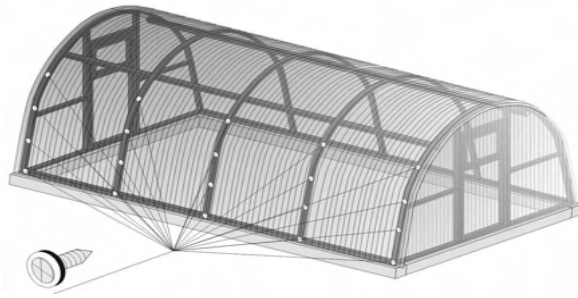
Pav. 10. Savisriegių varžtų tvirtinimo mazgai šiltnamio viršutinėje dalyje
